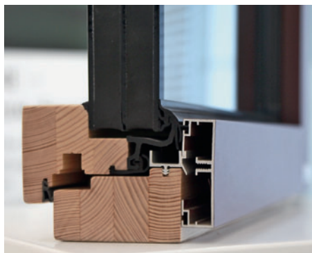
/ Im Querschnitt: Das Holz-Aluminium-Fenster Typ Slimline Ci-79 mit Dreifach-Verglasung.
