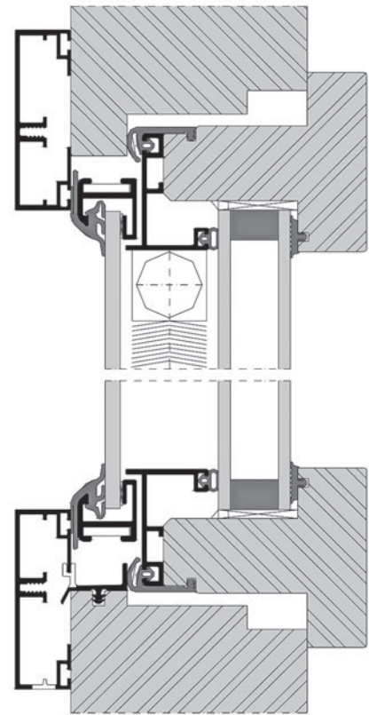
/ Das Holz/Aluminium-Fenster Slimline Cv-79 wurde zwischen den Scheiben mit einem Sonnenschutzsystem ausgestattet.
