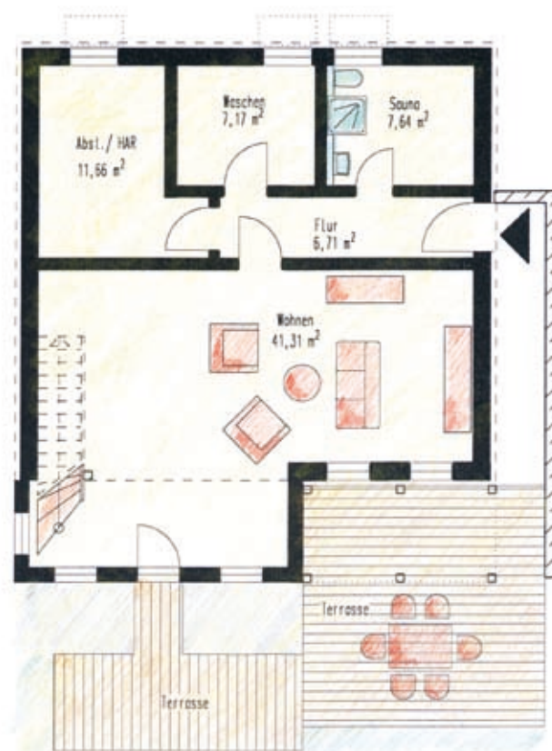
Gartengeschoß
